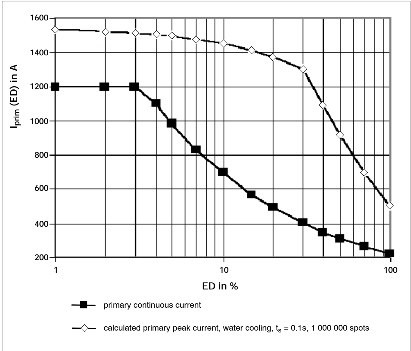
Load diagram, PSI 6200.XXX W1
