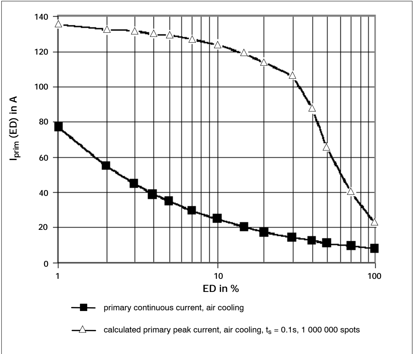
Load diagram, PSI 6025.XXX L1
